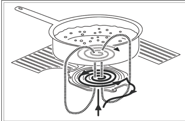
Funktionsprinzip und schematischer Aufbau eines Induktionskochherdes
